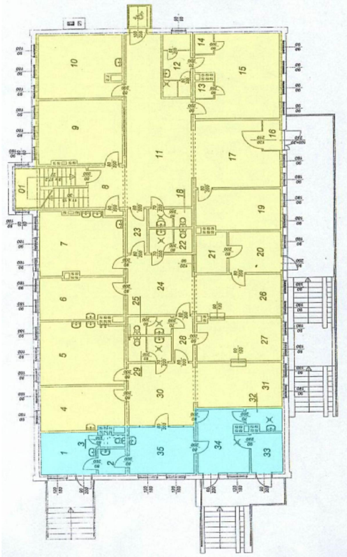
Przychodnia rejonowa, ul. Główna 28. Rzut parteru.
